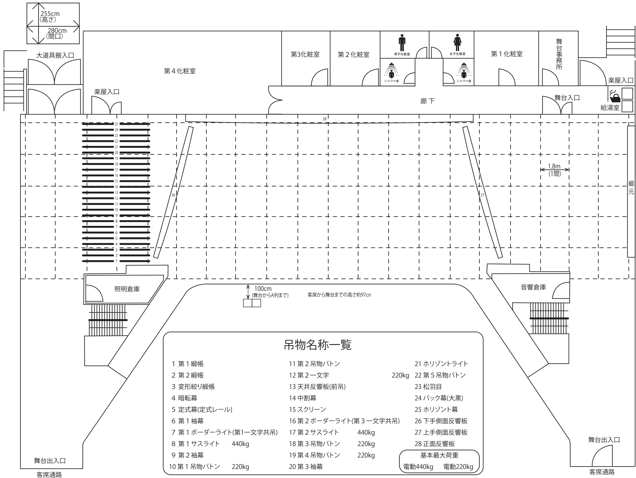
行田市産業文化会館ホール舞台平面図
